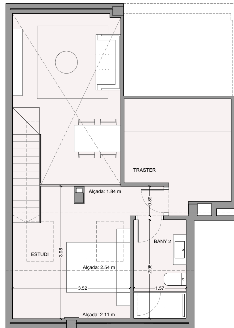
PG PLANTA GOLFES
