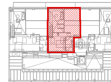
PG PLANTA GOLFES
