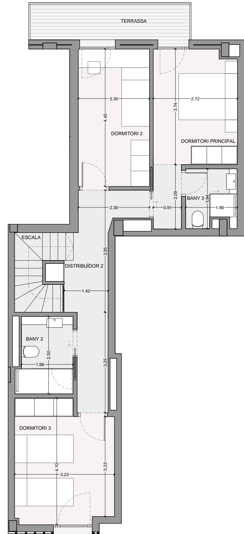
PB PLANTA BAIXA
